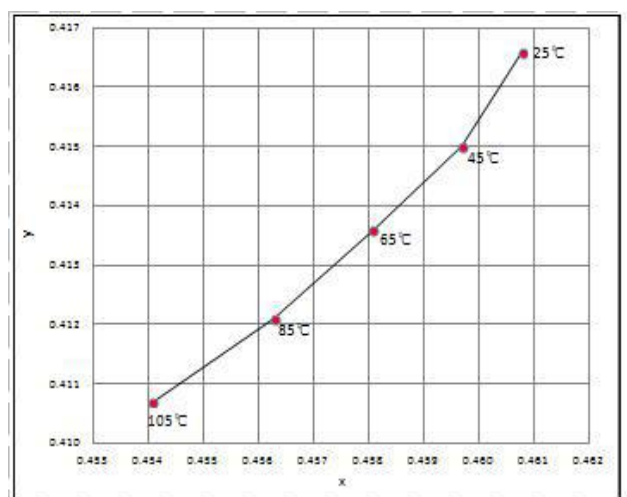
Fig 9. Ta vs. CIE x, y Shift
